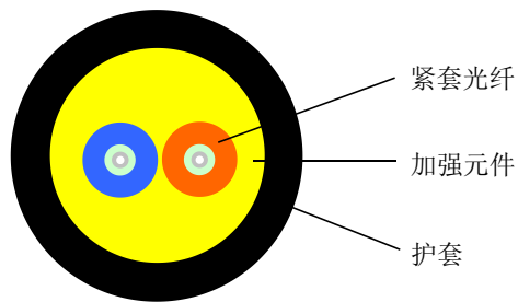
双芯圆形基站光缆III型
